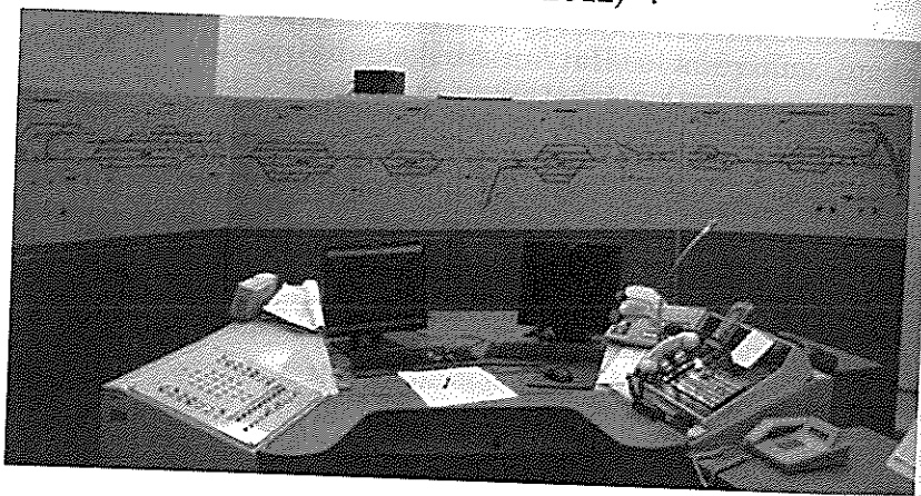
3. ábra A Mezőzombor–Nyíregyháza KÖFI-rendszer panorámatáblája. A hátsó falon láthatóak torzított méretekkkel a vasútvonal egyes állomásai. A közlekedő vonatokat színes lámpák jelentik vissza a kezelőnek. Az előtérben látható a kezelő munkahelye.
